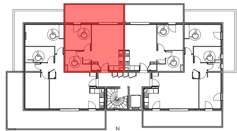
Plan d'étage courant R+1
